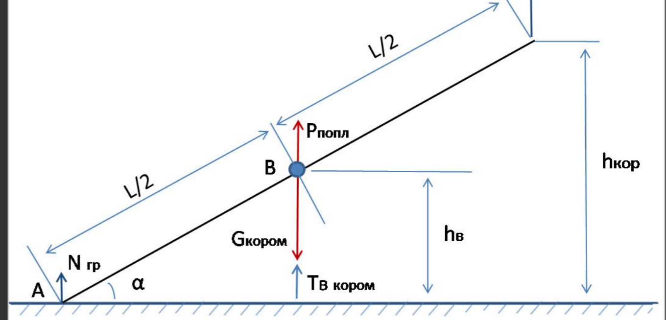
Рисунок 3 – Силы, действующие на коромысло в стоячей воде при поклевке
