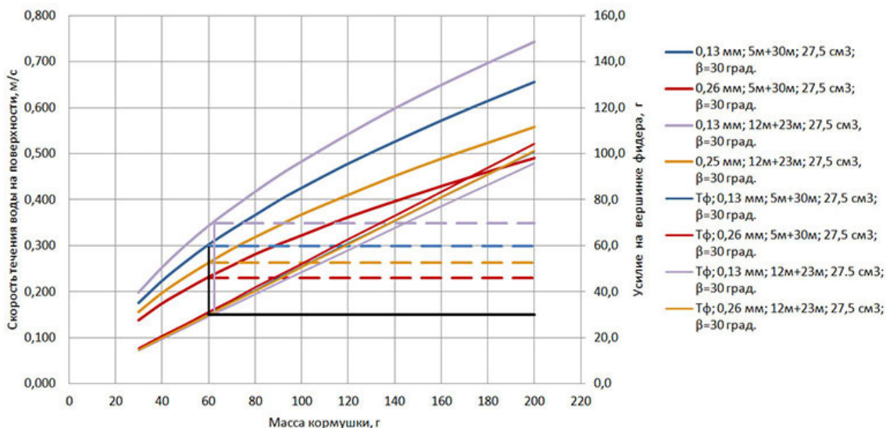
Рисунок 12 - Зависимость максимальной допустимой скорости течения воды на поверхности и усилий на вершинке фидера от массы кормушек при L_n + L_b = 5\text{ м} + 30\text{ м} и 12\text{ м} + 23\text{ м}
