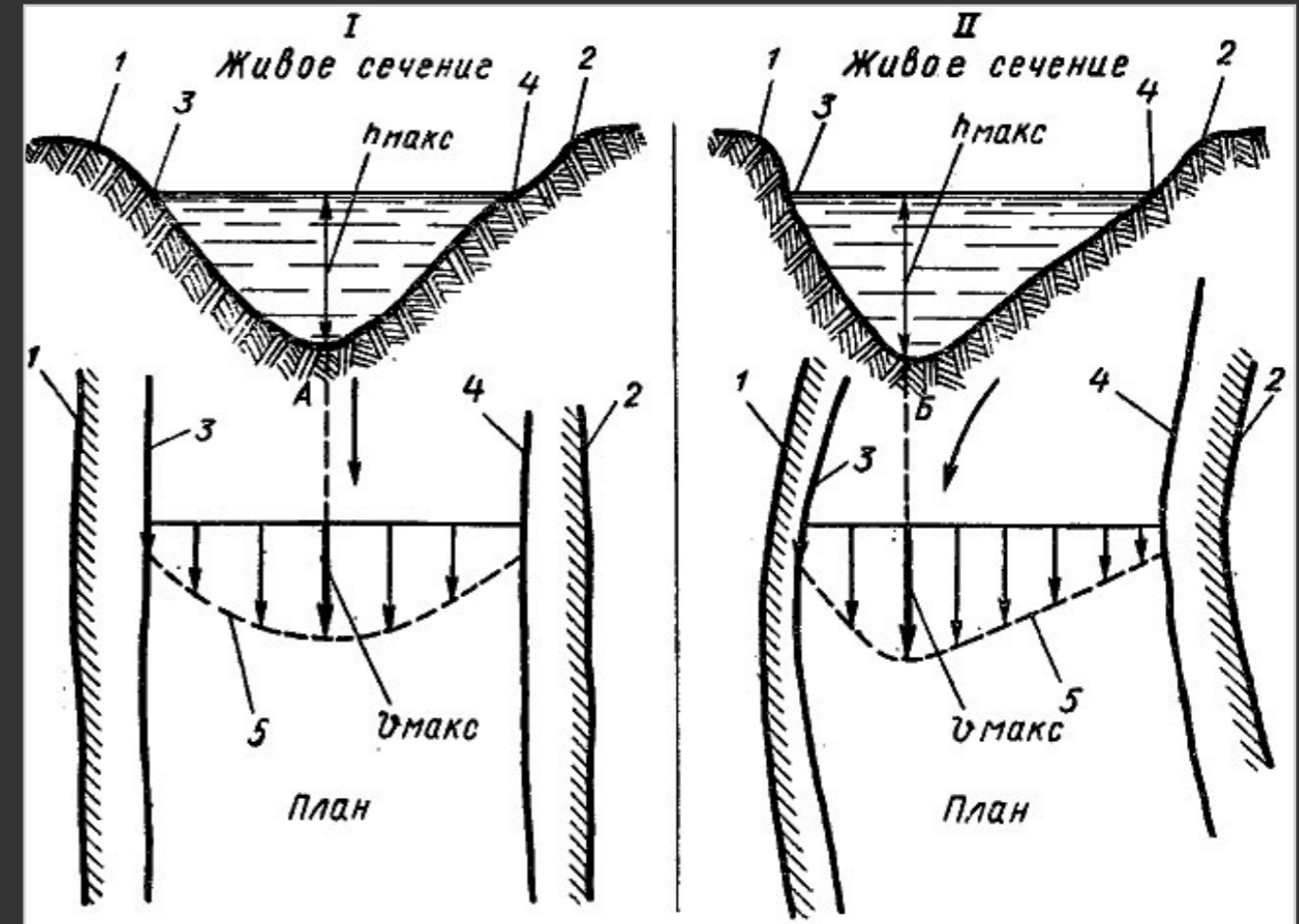
Рисунок 5 – Распределение поверхностных скоростей течения в плане: I — симметричное русло; II — несимметричное русло. 1 — бровка правого берега; 2 — бровка левого берега; 3 — правый урез воды; 4 — левый урез воды; 5 — распределение скоростей течения в плане
