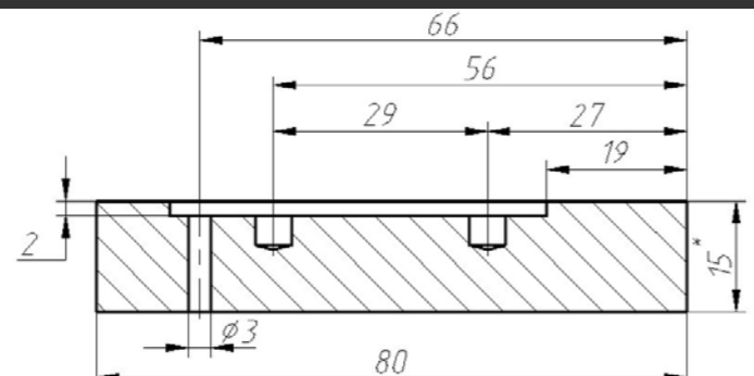
Рис. 3. Разрез
