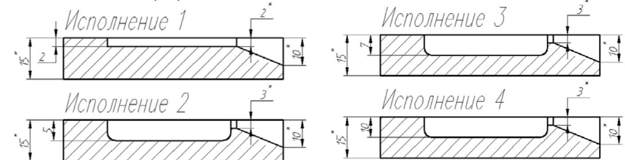
Рис.6. Нижняя часть, разрез
