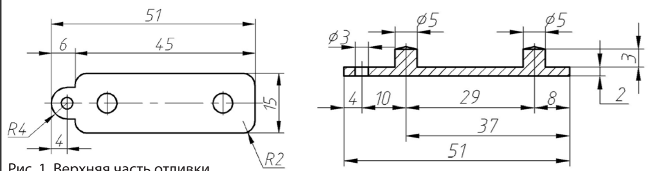
Рис. 1. Верхняя часть отливки
