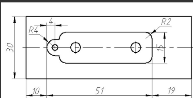
Рис. 2. Основание (верхняя крышка)
