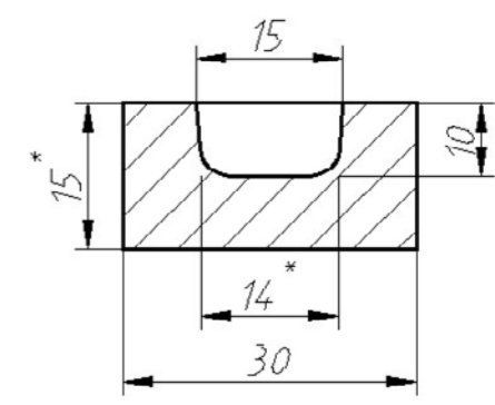
Рис. 5. Сечение
