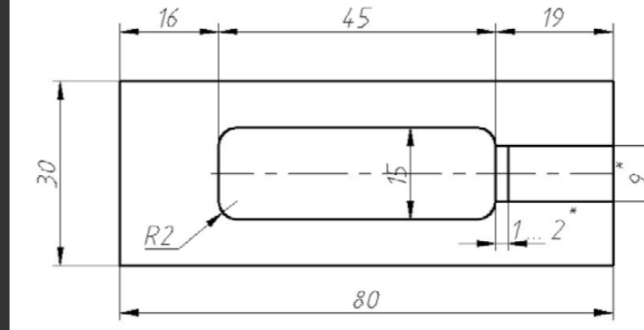
Рис. 4. Нижняя крышка
