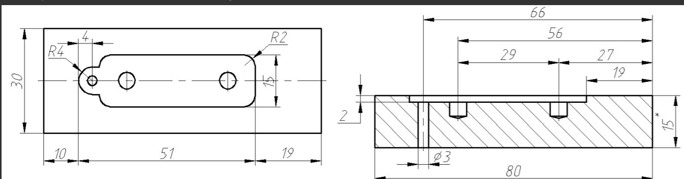
Рис. 2. Основание (верхняя крышка)
