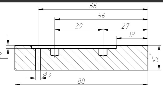
Рис. 3. Разрез
